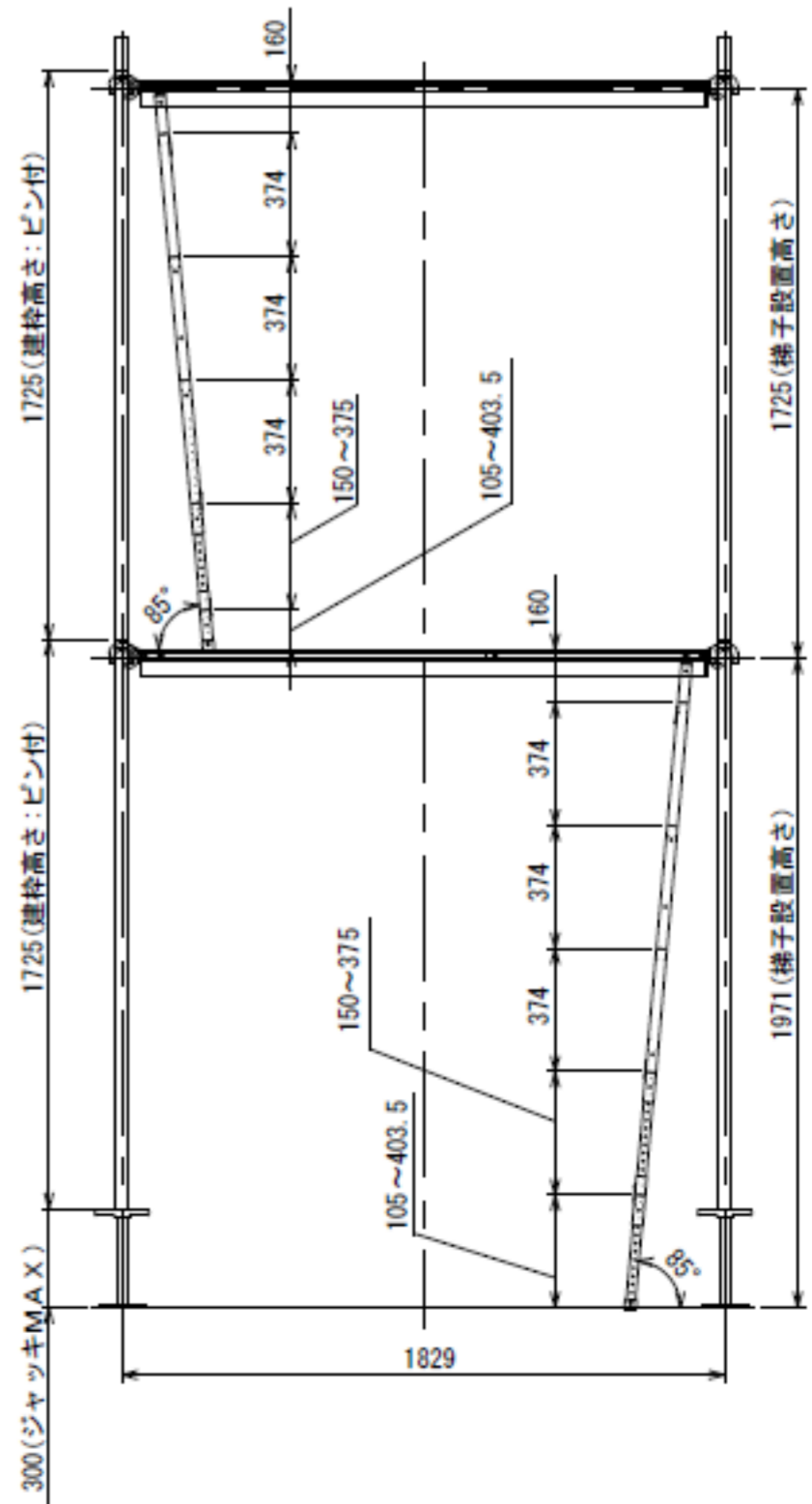
(枠組足場)
